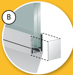
Detail B Basis detail bouwkundige aansluitingen 600 met eindkapje
